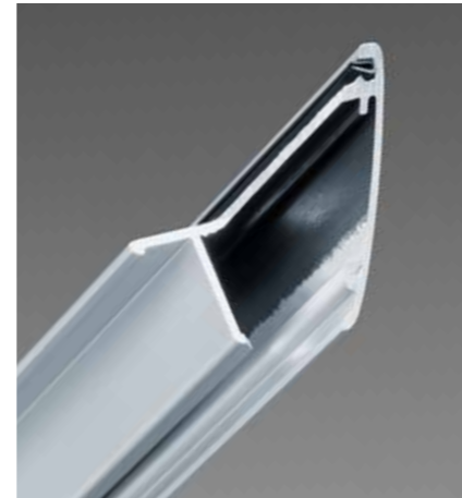
L'intérieur des profilés latéraux est entièrement peint en noir, afin d'éviter toute réflexion et d'assurer un obscurcissement complet.
